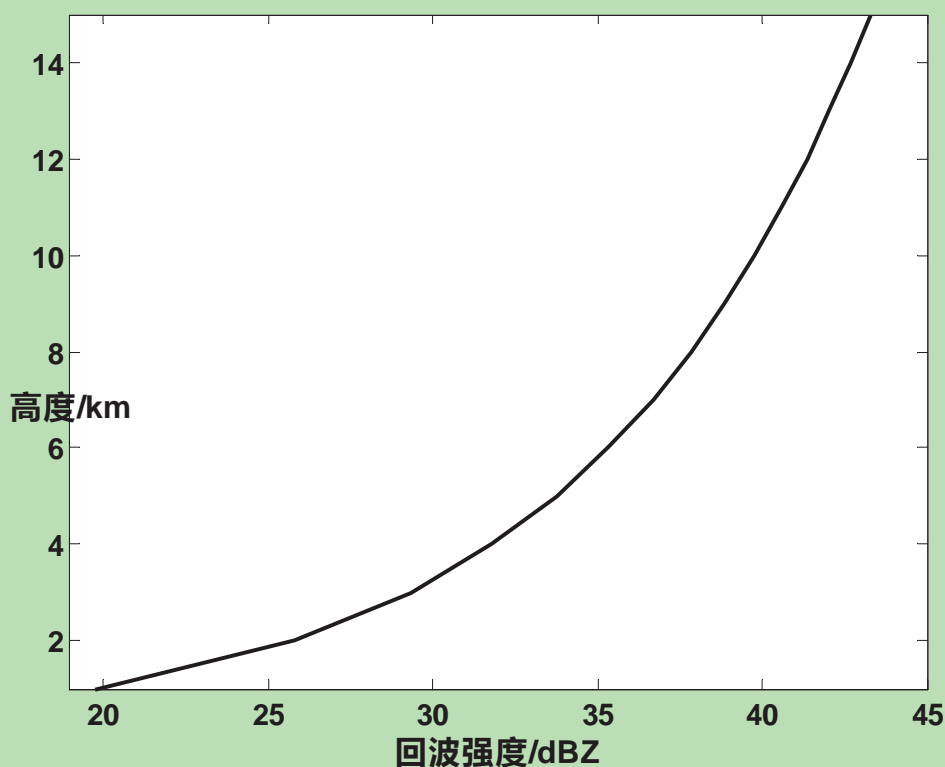
图 2 不同高度下雷达可测最大回波强度的垂直廓线图
